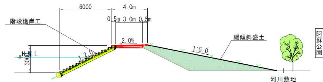
標準断面図
