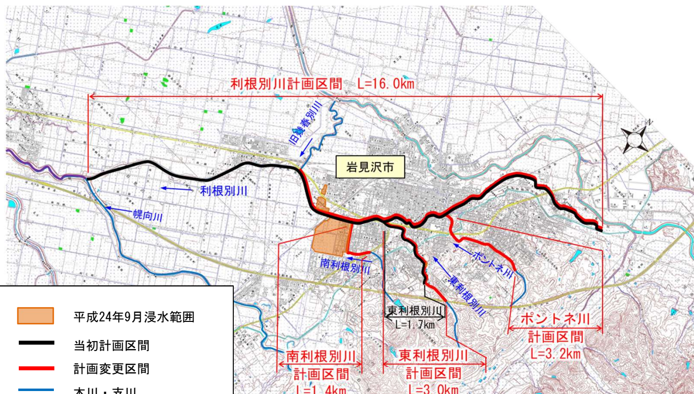
改修位置図
